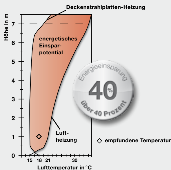
Abb. 2: Einsparpotenzial der Deckenstrahlplatten-Heizung gegenüber konventioneller Luftheizung bei gleicher empfundener Temperatur.
