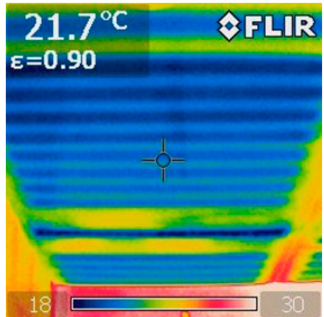
Abb. 3: Infrarotaufnahme einer Klimadecke in Kühlfunktion
