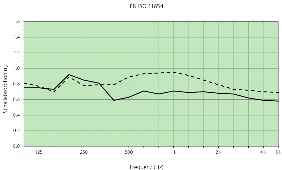
Abb. 6: Schallabsorptionskurve über verschiedene Frequenzen am Beispiel einer Klimadecke aus Metall:
