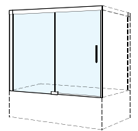
Kombination mit Seitenwand En combinaison avec paroi latérale
