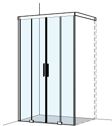
Kombination mit Seitenwand En combinaison avec paroi latérale
