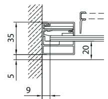
Montage bodeneben Montage à fleur de sol
