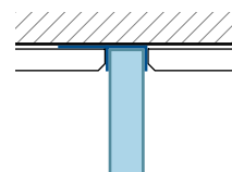
Wandprofil UP Profil mural encastré
