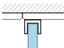
Wandprofil AP Profilo a posa sporgente
