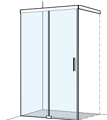
Kombination mit Seitenwand festelementseitig Combinazione con parete laterale lato elemento fisso
