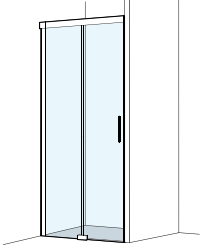
Kombination mit Seitenwand türseitig Combinazione con parete laterale lato porta
