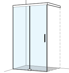
Kombination mit Seitenwand festelementseitig Combinazione con parete laterale lato elemento fisso
