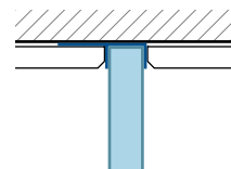
Wandprofil UP Profilo a posa incassata
